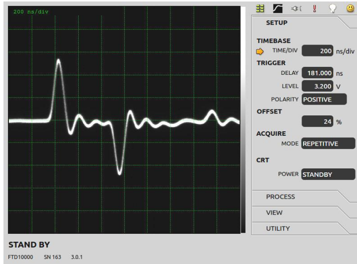
Local GUI
